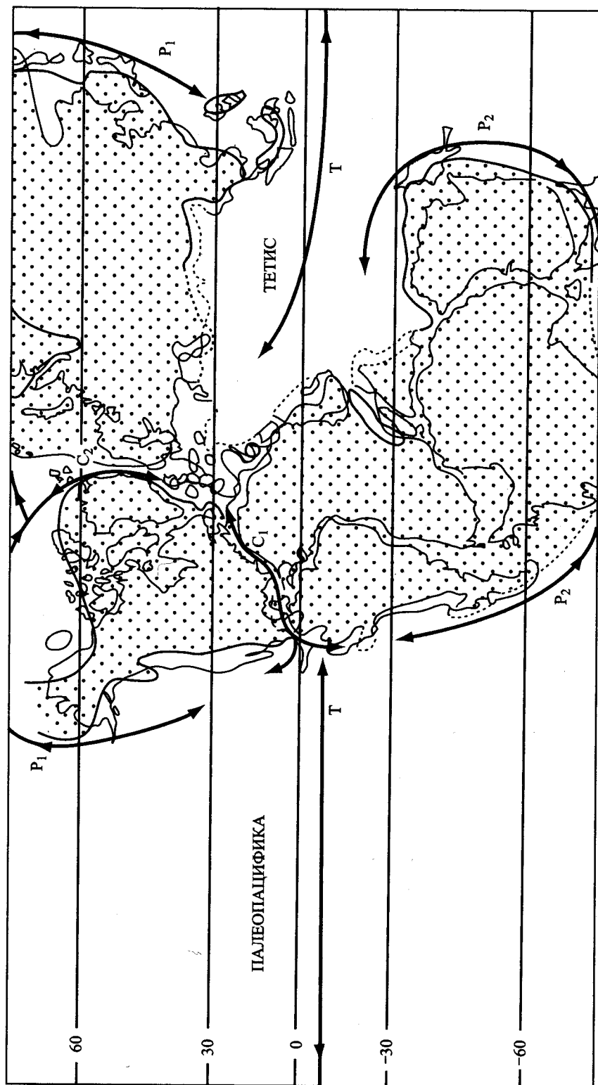
Рис. 5. Глобальная палеогеографическая реконструкция для раннеюрского времени (плинсбах) с указанием возможных путей миграции морских организмов
